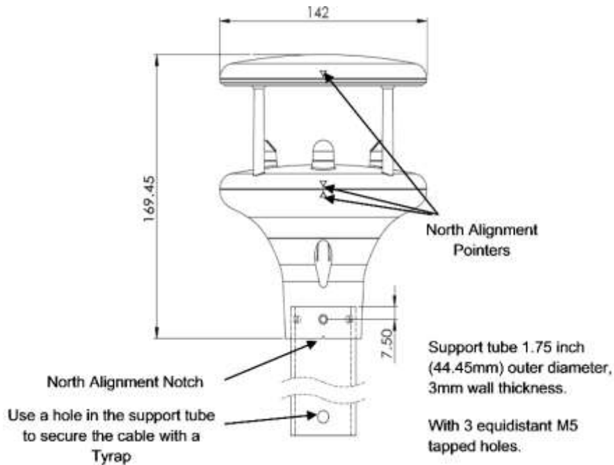
GMX200
